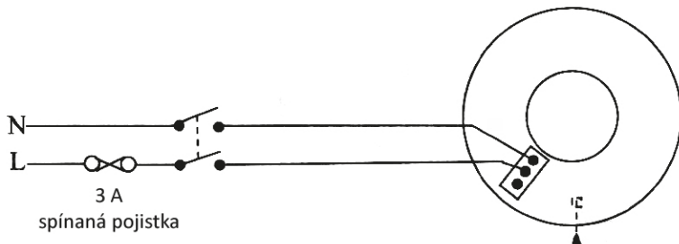
Schéma zapojení - ventilátor s modulem bez externího vypínače (Ize doporučit s moduly PCM, HTM, PRTM a PRHTM)
