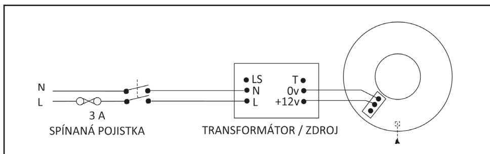
Schéma zapojení - ventilátor 12 VDC s modulem bez externého vypínače (Ize doporučit s moduly PCS, DTS, HTS, PRTS a PRHTS)
