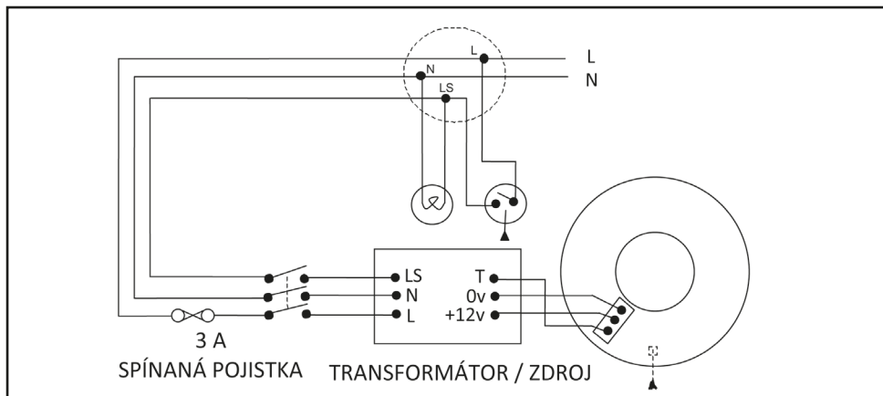
Schéma zapojení - ventilátor 12 VDC s modulem s externím vypínačem (Ize doporučit s moduly PCTS, DTS, HTS)
